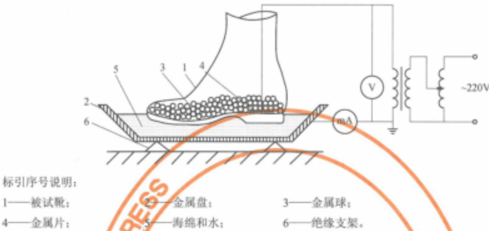
图 D.7 辅助型绝缘靴工频耐压及泄漏电流试验接线图
