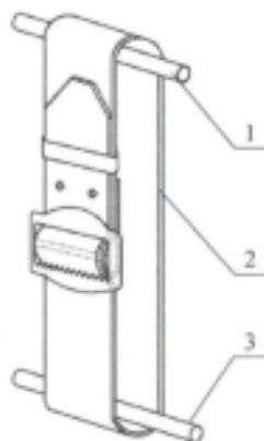
图 C.9 登杆脚扣静负荷试验示意图
